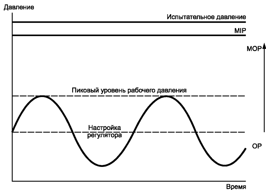
Рисунок 1. Соотношение давлений
